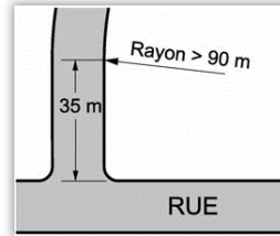
Croquis 4.9 Aménagement d'une courbe à proximité d'une intersection
