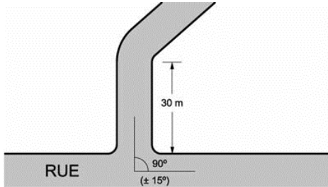
Croquis 4.6 Aménagement d'une intersection
