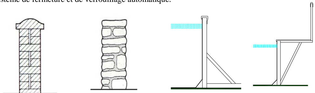
muret non escaladable muret non escaladable étais escaladables étais non escaladables
