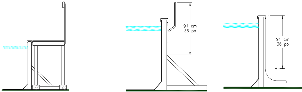
étais surmontés d'une plate-forme étais surmontés d'un garde-corps substitution des étais
